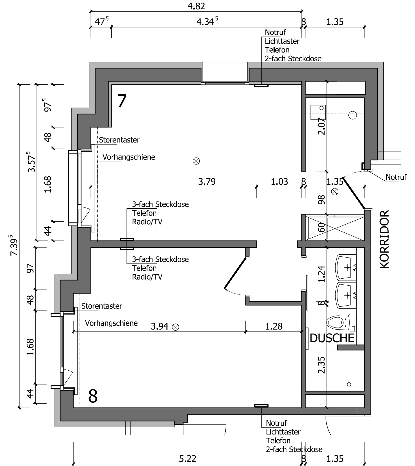
ZIMMERGRUNDRISS MST 1:50
